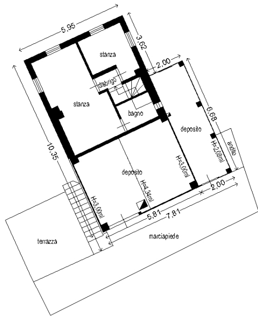
PIANO PRIMO h=2,55ml
